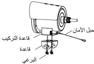
الشكل 1-8 تثبيت الكاميرا على القاعدة
