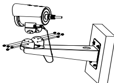
Gambar 1-6 Memasang Braket Pemasangan di Dinding
