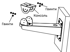
Рисунок 1-7. Зніміть консоль
