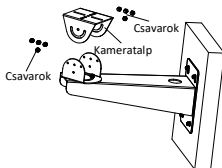
1-7. ábra: A kameratalp eltávolítása
