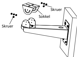
Figur 1-7 Fjern soklen
