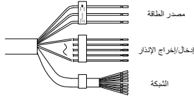
الشكل 1-5 نظرة عامة على الكابلات
