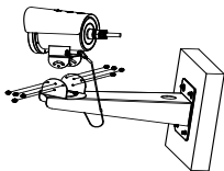
Afbeeldingen 1-6 De muurmontagebeugel monteren
