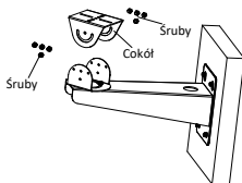
Rysunek 1-7 Odłączanie cokołu
