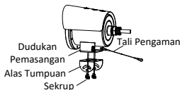
Gambar 1-8 Memasang Kamera ke Alas Tumpuan
