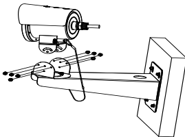
Figura 1-6 Instalação do suporte de montagem em parede
