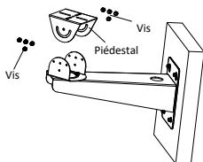
Figure 1-7 Retrait du piédestal
