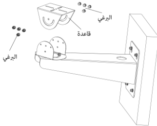
الشكل 1-7 إزالة القاعدة
