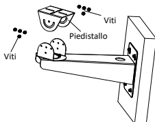
Figura 1-7 Rimuovere il piedistallo
