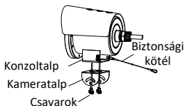
1-8. ábra: A kamera rögzítése a kameratalphoz
