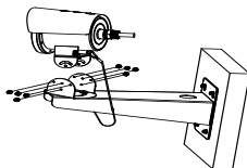
Rysunek 1-9 Dostosowanie kąta obrotu
