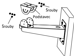
Obrázek 1-7 Demontáž podstavce
