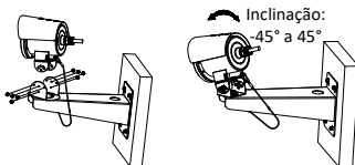
Figura 1-10 Fixação da câmara ao suporte de montagem em parede
