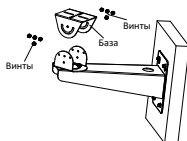
Рис. 1-7 Снятие базы
