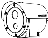
Рис. 1-3 Общий вид взрывозащитной сетевой цилиндрической камеры (1)
