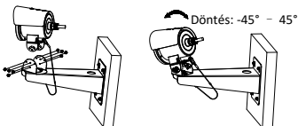
1-10. ábra: A kamera rögzítése a fali konzolra
