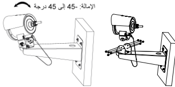
الشكل 1-10 تأمين الكاميرا على حامل التثبيت على الجدار
