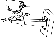
Şekil 1-6 Duvara Montaj Braketinin Takılması
