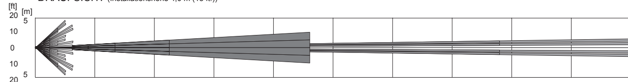
DRAUFSICHT (Installationshöhe 4,0 m (13 ft.))
