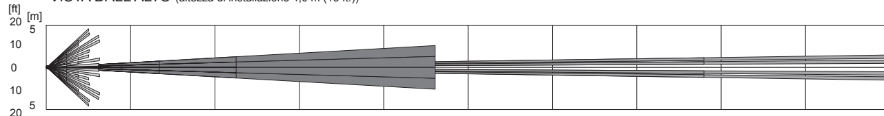
VISTA DALL'ALTO (altezza di installazione 4,0 m (13 ft.))
